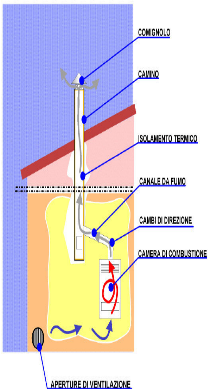
IMPIANTO A CONDOTTO SINGOLO
