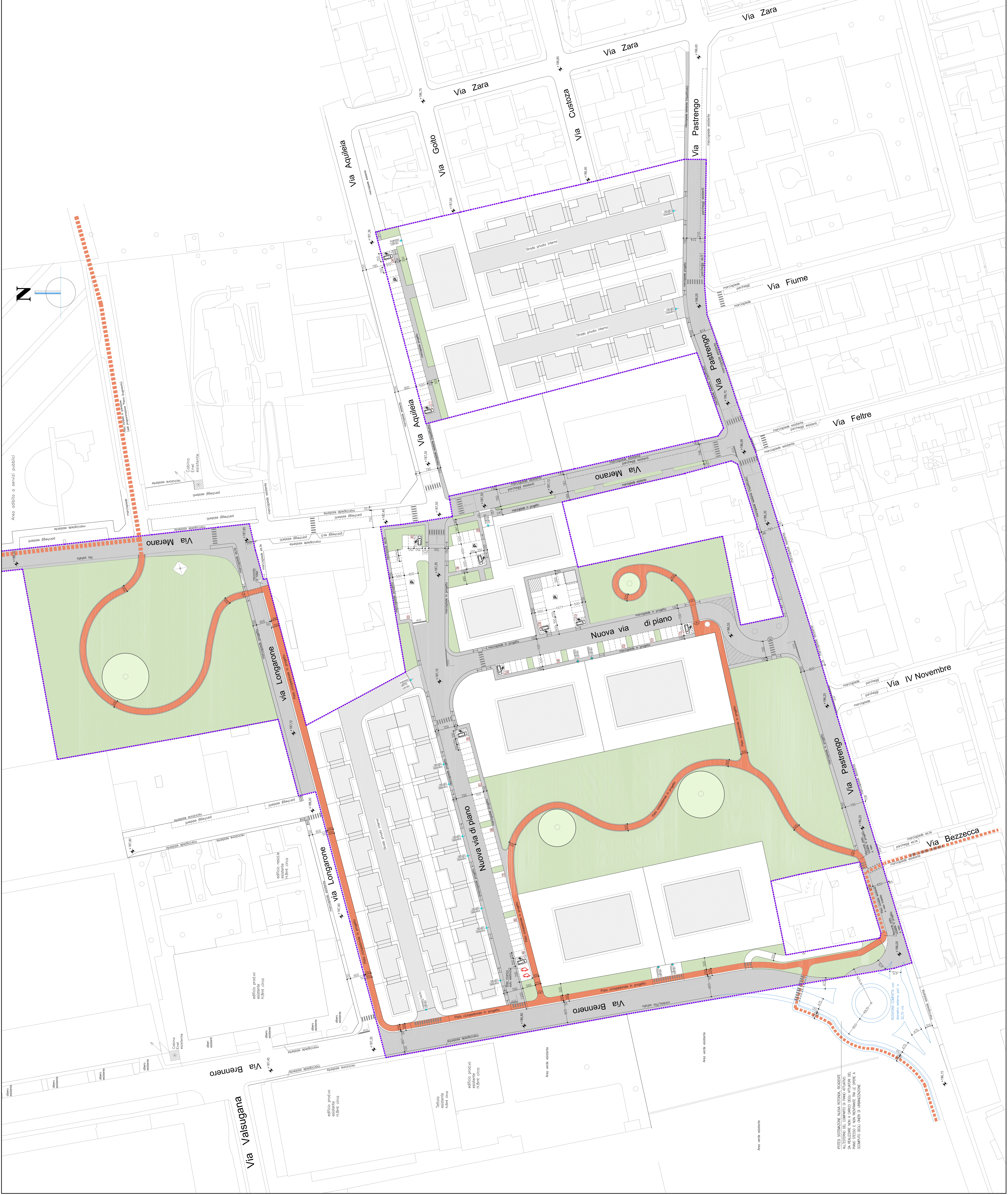
PORZIONE "B" - VIABILITÀ VEICOLARE
